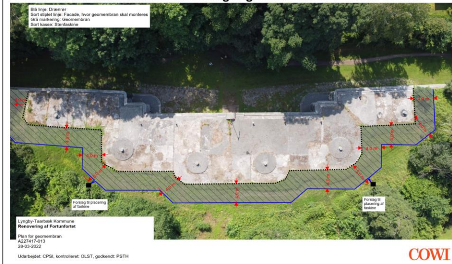
Luftfoto af Fortunfortet med markering af geomembran i 4 meters bredde
