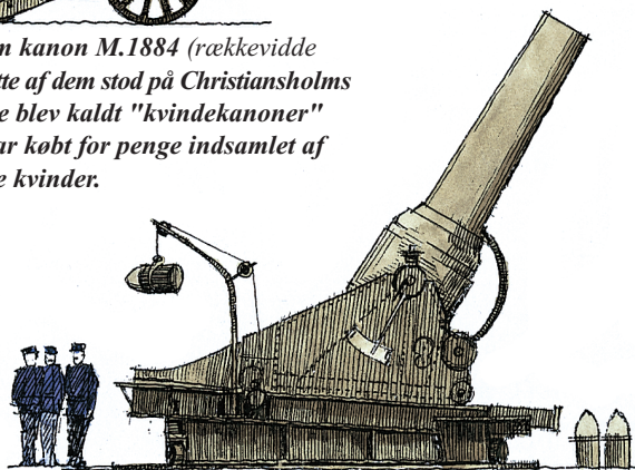
29 cm haubitze M 1874/1910 (rækkevidde 10,3 km). Står på Charlottenlund Fort.
